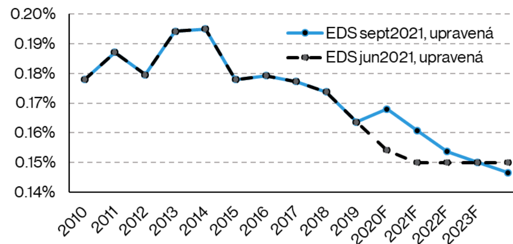
Očistená EDS
